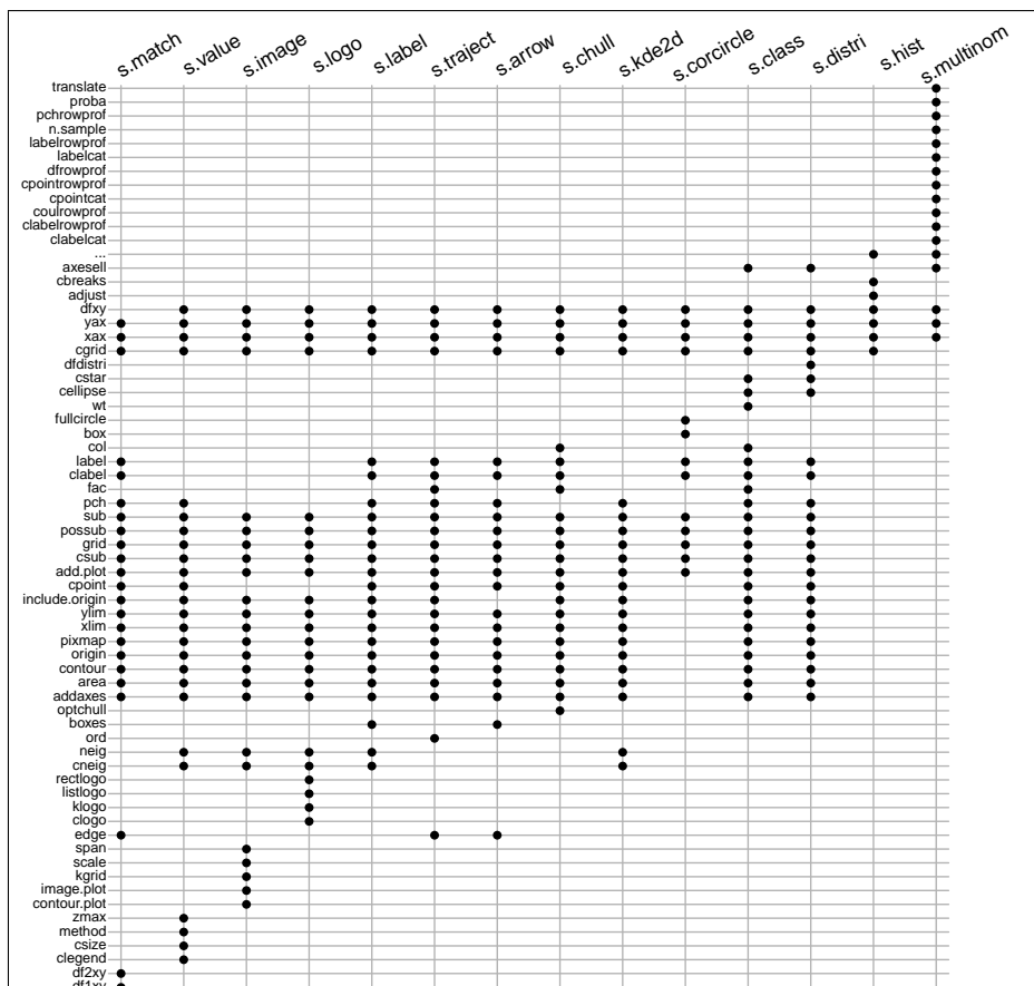
FIG. 1 – Présentation synthétique des arguments disponibles pour les fonctions de la famille s.* . Les 66 arguments possibles sont disposés en ligne, les 14 fonctions de la famille s.* sont disposées en colonne. Un point de coordonnées (i, j) signifie que l'argument i est explicitement disponible pour la fonction j . L'ordre des lignes et des colonnes est selon le premier facteur de l'AFC de cette table de présence/absence. La fonction s.multinom() se démarque par le nombre d'arguments qui lui sont spécifiques. Les fonctions s.match() , s.value() , s.image() et s.logo() se distinguent par leur arguments additionnels. On note quatre arguments quasi-ubiquistes ( viz dfxy , yax , xax et cgrid ) ainsi qu'un noyau d'arguments très utilisés au milieu de la table. L'étude détaillée de la fonction s.label() permettra de couvrir les arguments les plus usuels.
