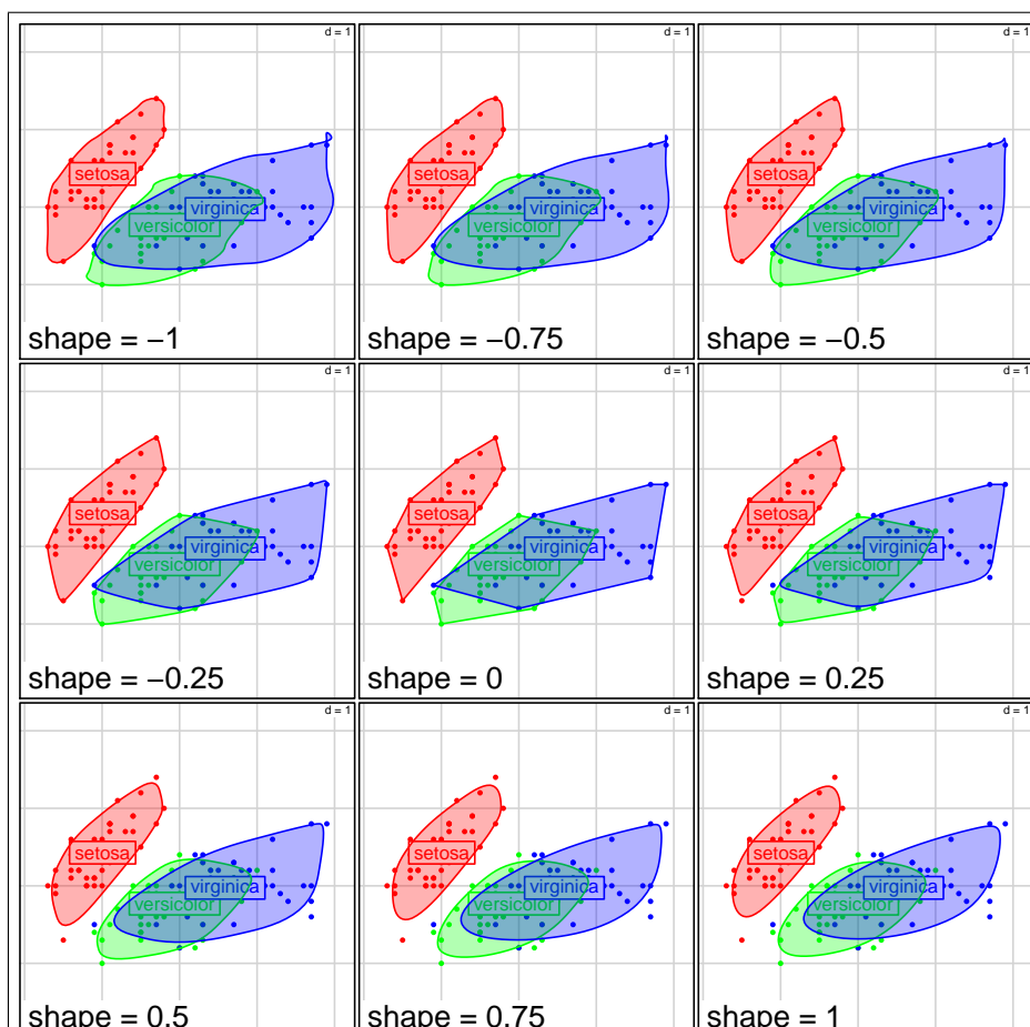
FIG. 2 – Démonstration de l'effet du paramètre shape de la fonction standard xspline() sur l'aspect des patatoïdes représentant des classes de points. Avec shape = 0 on retrouve au centre le rendu de s.chull(optchull = 1) . Attention : l'utilisation ici de couleurs semi-transparentes pour le remplissage des patatoïdes n'est pas supportée par tous les périphériques graphiques.
